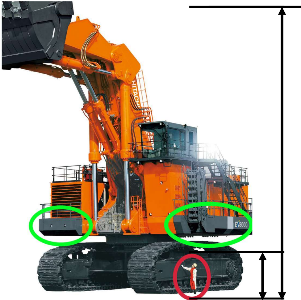
油圧ショベル フェンダー 一般男性1.7mに対し、10m超の 機体に搭載されています
